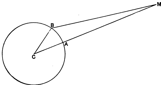
FIG. 31.—Parallax
