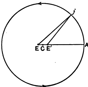
FIG. 35.—The equant.
